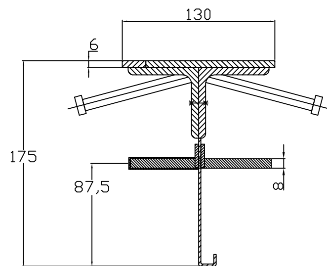
CONECTO SINUS 06NCE130-5D-T8 h=175 Section
