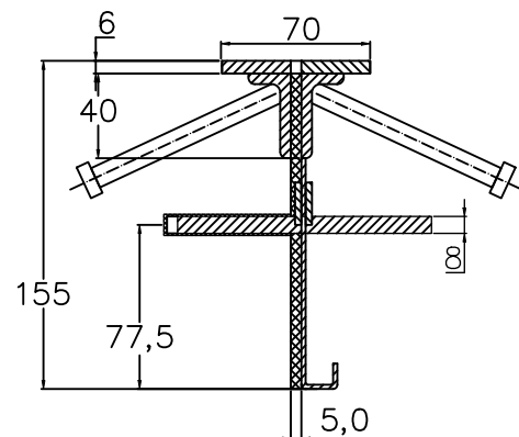
CONECTO SINUS 06NCC65/40x20-5D-T8 h=155 Section
