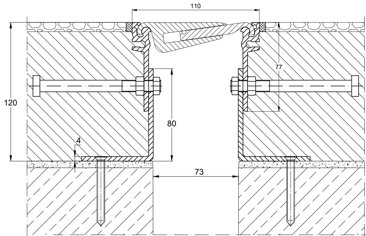
CONECTO AL 110.15.120& SECTION
