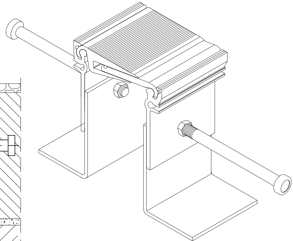
CONECTO AL 110.15.120& VIEW
