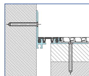
Eckprofil
