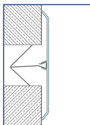
Deckenprofil, Aufsatz
