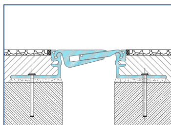
Flächenbündige Ausführung
