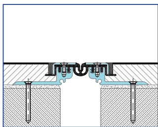
Flächenbündige Ausführung
