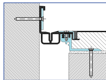
Eckprofil
