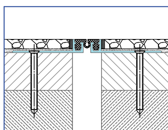
Flächenbündige Ausführung
