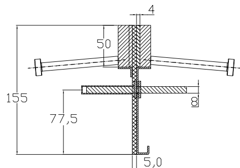
CONECTO SINUS 04NS50-4D-T8 h=155 SECTION
